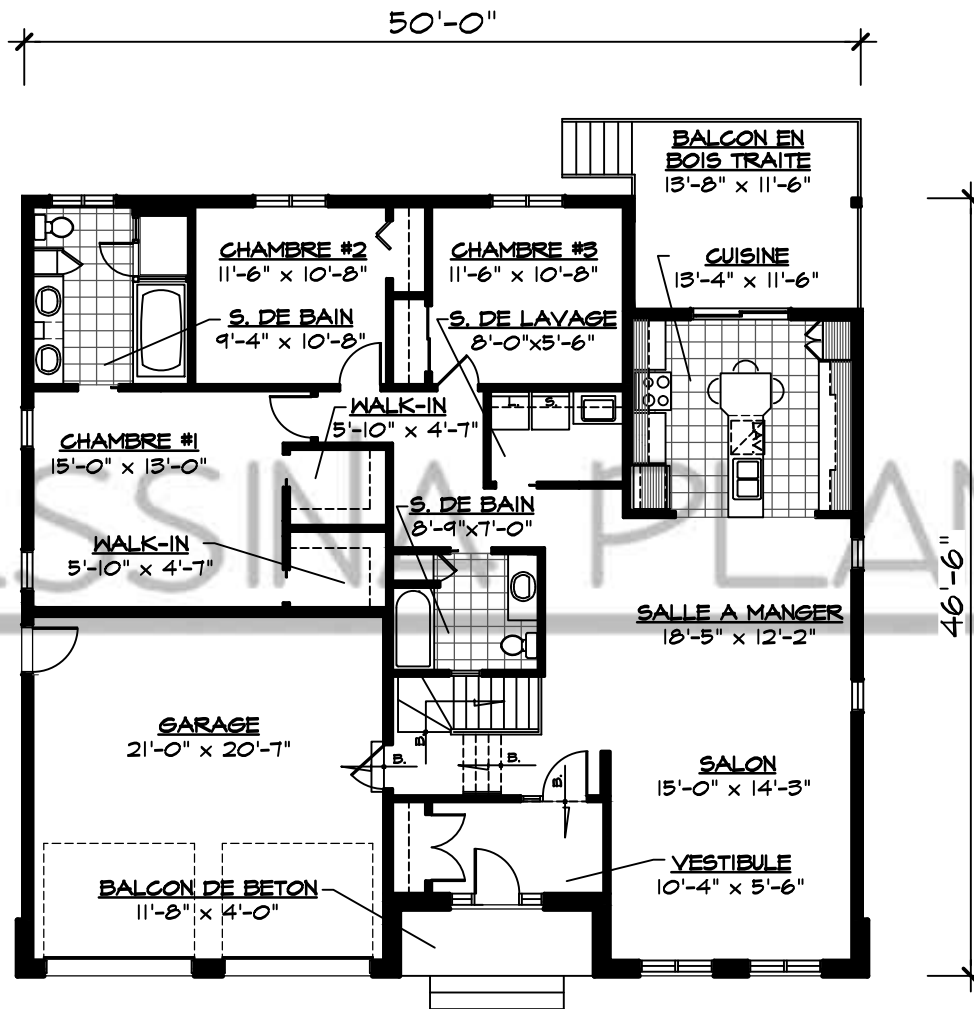
PLAN DU REZ-DE-CHAUSSEE SUP.: 1701 pi.ca. + GARAGE 487 pi.ca.
